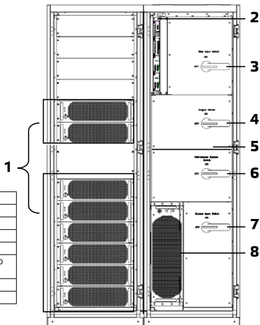
Рис. 2-14. Вид ИБП мощностью 400 кВА (расширенный) с открытой передней дверцей
