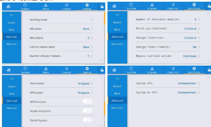
о Рис. 3-30. Интерфейс расширенных параметров
