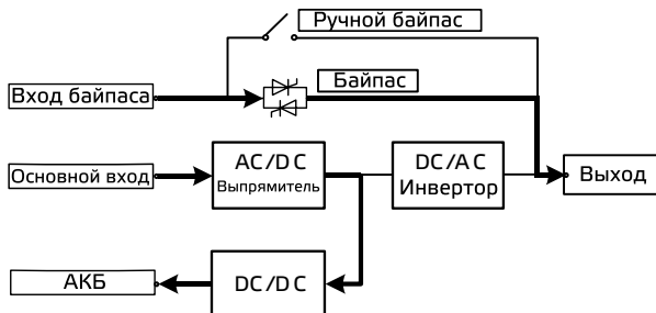
Рис. 2-3. Принципиальная схема режима байпаса
