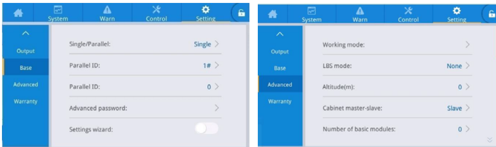
Рис. 4-8. Интерфейс настройки параллельных параметров
