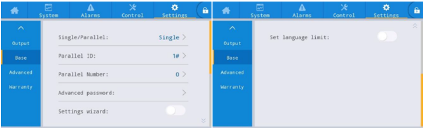
Рис. 3-29. Интерфейс основных параметров
