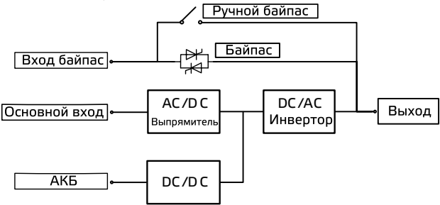
◦ Рис. 2-1 Функциональная схема
