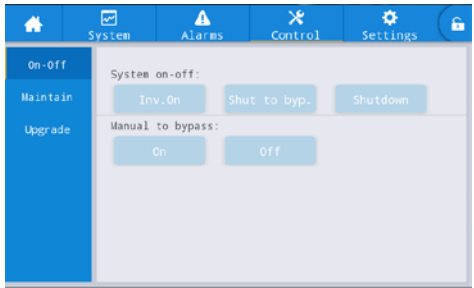
Рис. 3-18. Интерфейс «Вкл/Выкл»
