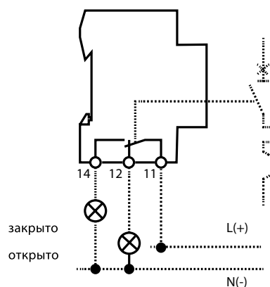
Схема подключения
