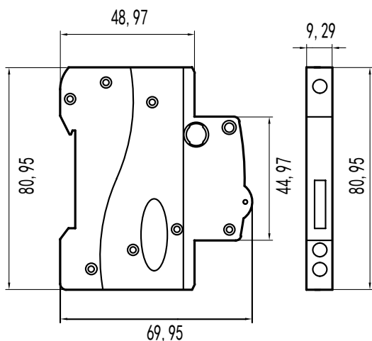
Габаритные размеры
