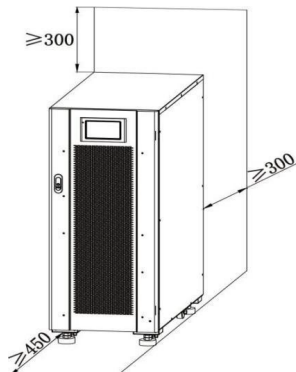
Рис. 3 – 1 Отступы от ИБП мощностью 80 кВА (единицы измерения: мм)
