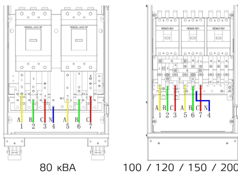
Рис. 3 – 10 Подключение входного кабеля переменного тока
