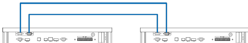
Рис. 3 – 15 Схема соединения кабелей управления параллельной системы 1+1
