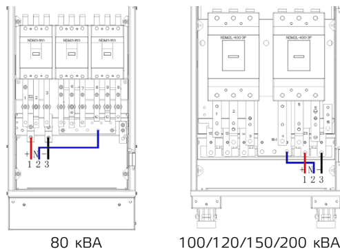
Рис. 3 – 9 Подключение кабелей аккумуляторов
