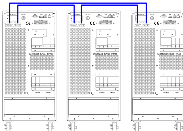
Рис. 5–6 Параллельное соединение
