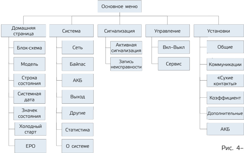
Рис. 4-2 Меню
