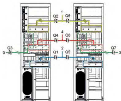
Рис. 2-48 Схема подключения параллельной системы 1+1 (500 кВА)
