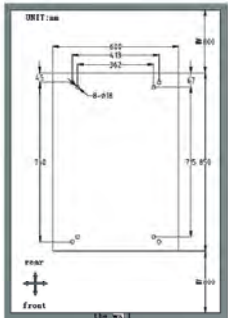
Рис. 2-9 Маркировка для 200 кВА и 300 кВА
