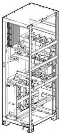
Рис. 2-26 Нижний путь прокладки сигнального кабеля (500 кВА)
