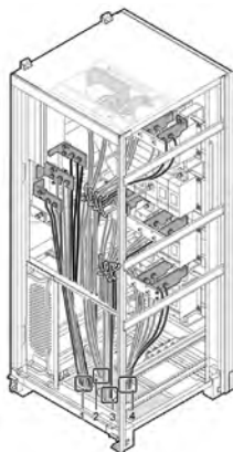
Рис. 2-24 Нижняя прокладка и места крепления силовых кабелей (500 кВА)
