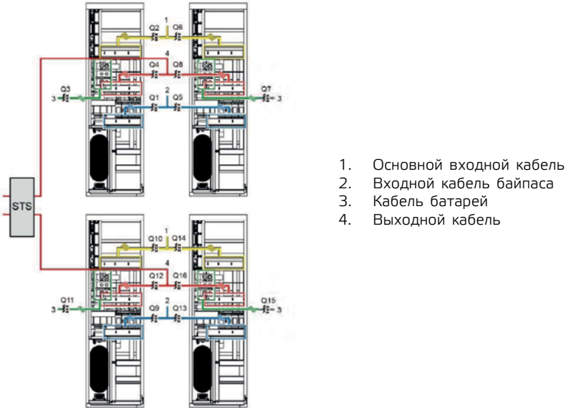
Рис. 2-50 Схема электропроводки параллельной системы с двумя шинами (500 кВА)
