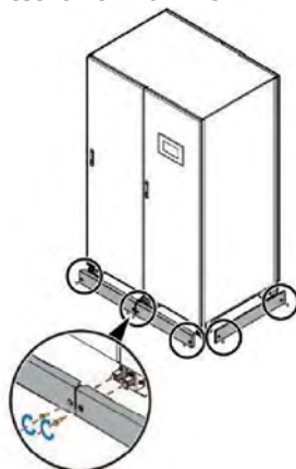
Рис. 2-13 Установка передних и задних перегородок
