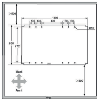
Рис. 2-55 Размер установочных отверстий антисейсмического узла (600 кВА, единица измерения: мм)
