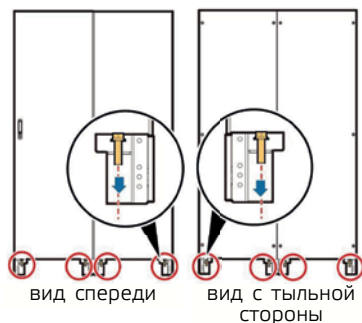
Рис. 2-12 Установка дюбеля
