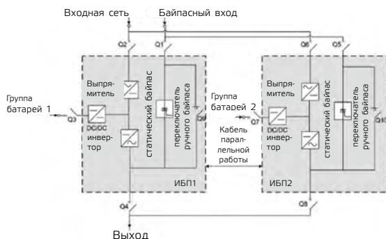
Рис. 2-47 Функциональная блок-схема 1+1 и схема соединений параллельной системы 1+1
