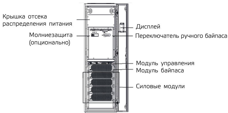
Рис. 1-4 Структура ИБП 200 кВА (стандартная)
