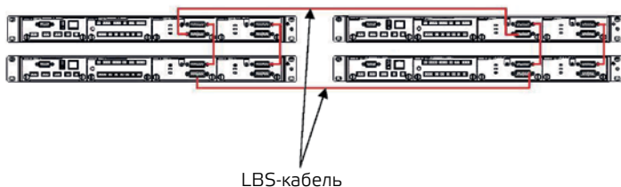
Рис. 2-52 Подключение кабеля управления для параллельной системы с двойной шиной
