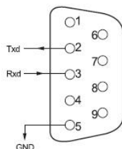
Порт RS232 (COM-port).
