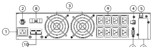
ИБП 2 кВА (48 В), 2 кВА (72 В) и 3 кВА (72 В)
