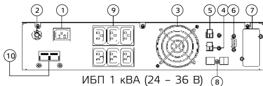
ИБП 1 кВА (24 – 36 В)
