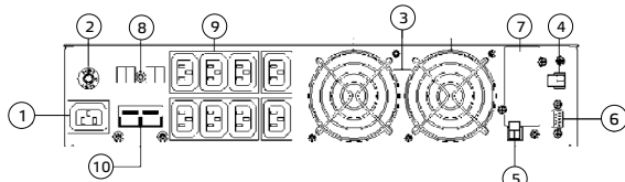
ИБП 2 кВА (96 В) и 3 кВА (96 В)
