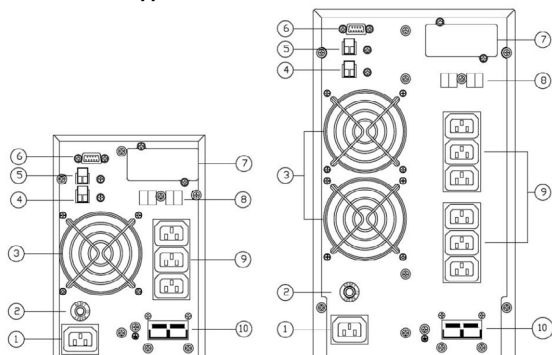
ИБП 1 кВА
