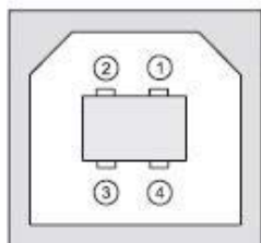
Порт USB
