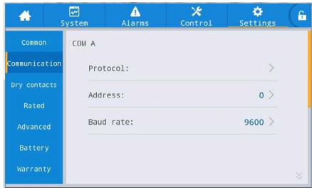
Рис. 4 – 15 Интерфейс настроек связи
