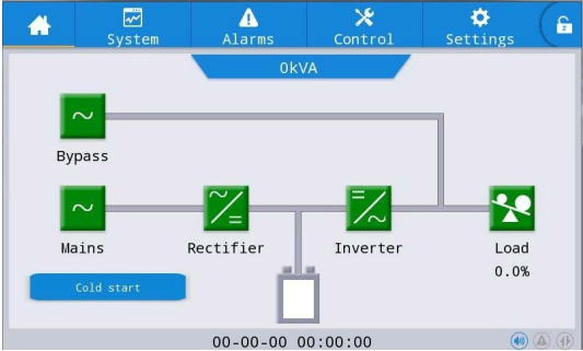
Рис. 5 – 1 Кнопка холодного запуска на ЖК-дисплее
