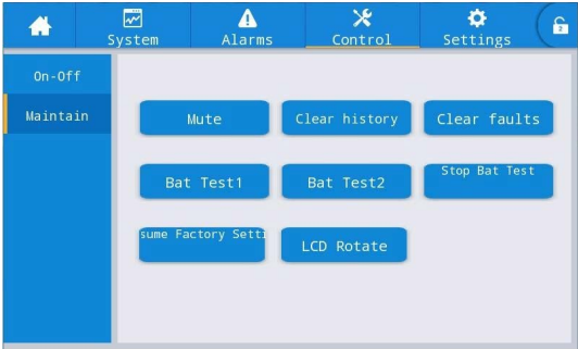
Рис. 5 – 4 Страница обслуживания батарей
