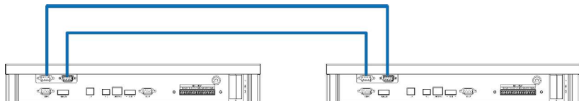
Рис. 3 – 15 Схема соединения кабелей управления параллельной системы 1+1
