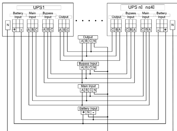
Рис. 3 – 14 Схема силовой проводки параллельной системы
