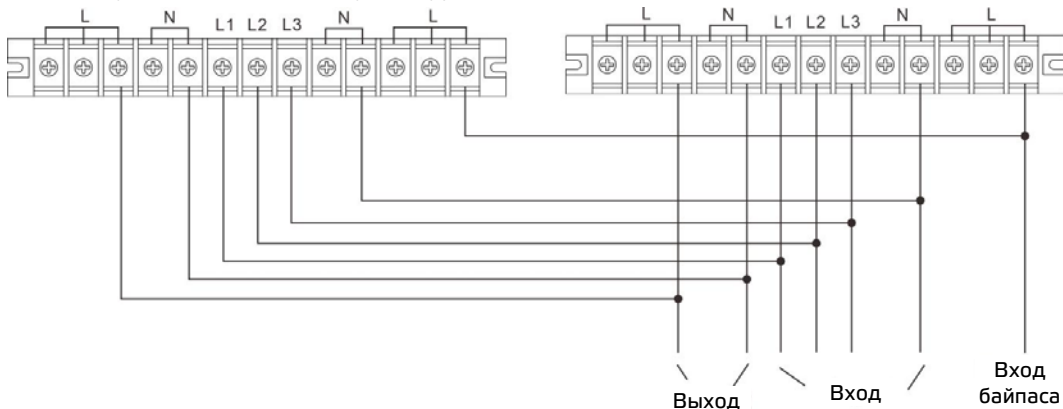
Схема подключения параллельной системы для 3:1 10К / 15К / 20К
