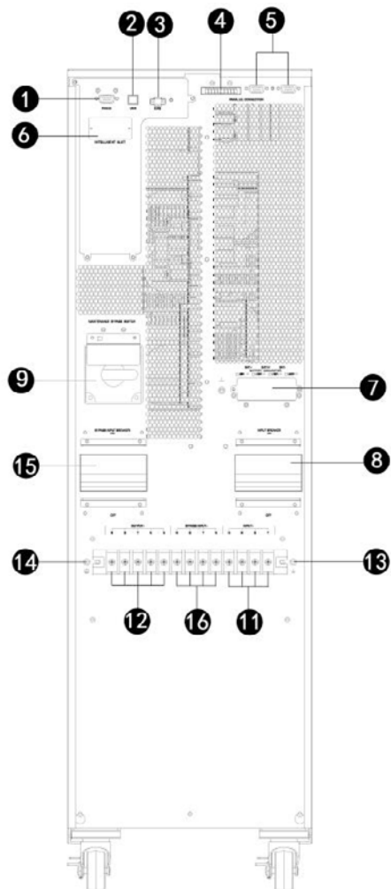
30K / 40K Задняя панель
