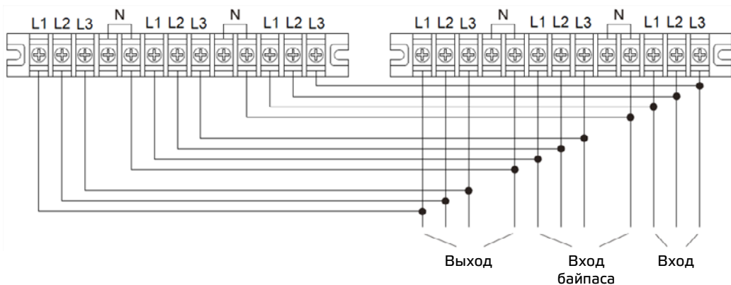
Схема подключения параллельной системы для 3:3 30К / 40К
