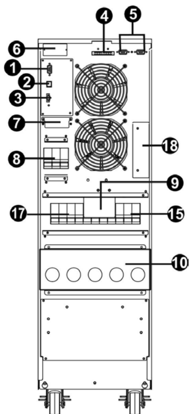
10K / 15K / 20K Задняя панель
