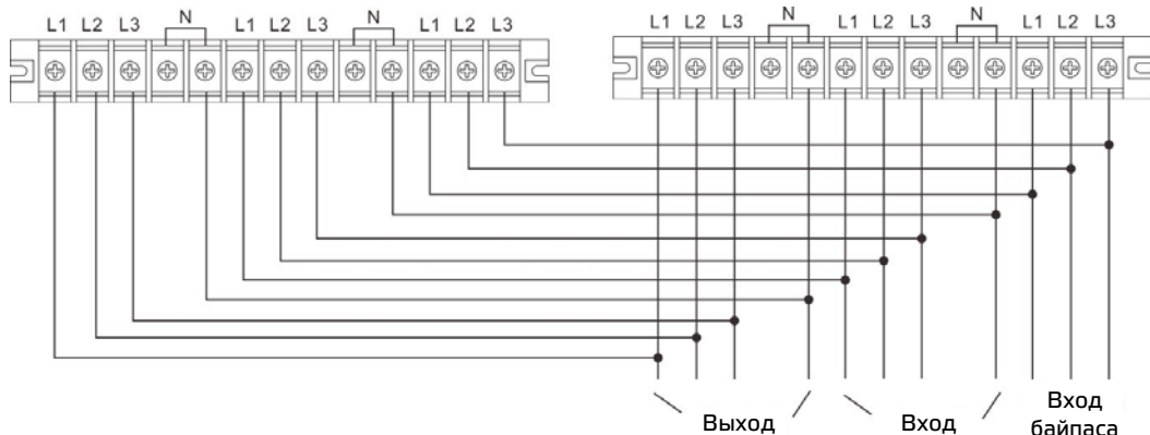
Схема подключения параллельной системы для 3:3 10К / 15К / 20К
