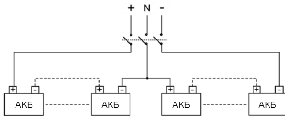
Рис. 3–2 Схема электропроводки аккумуляторной группы
