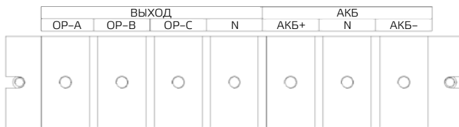
Рис. 3-4 (b) Клеммы подключения в модели 30 кВА
