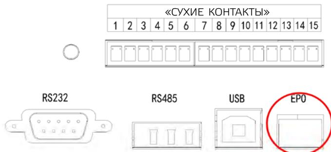
Рис. 5–4 Порт EPO в интерфейсе связи
