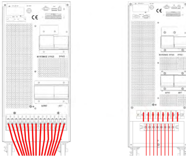
Рис. 3–3 Кабельный ввод
