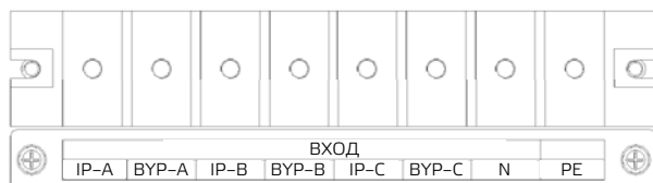
Рис. 3-5 Клеммы подключения в моделях 40-60 кВА
