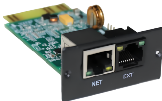
Общий вид (карта расширения) Размеры: 77 x 51.8 x 25.8 mm
