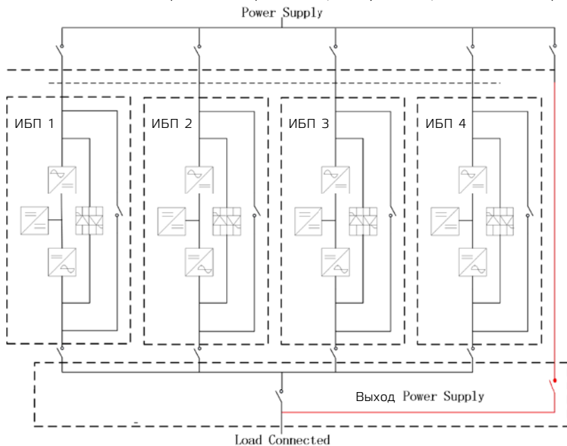
Рис. 5–5 Параллельная схема
